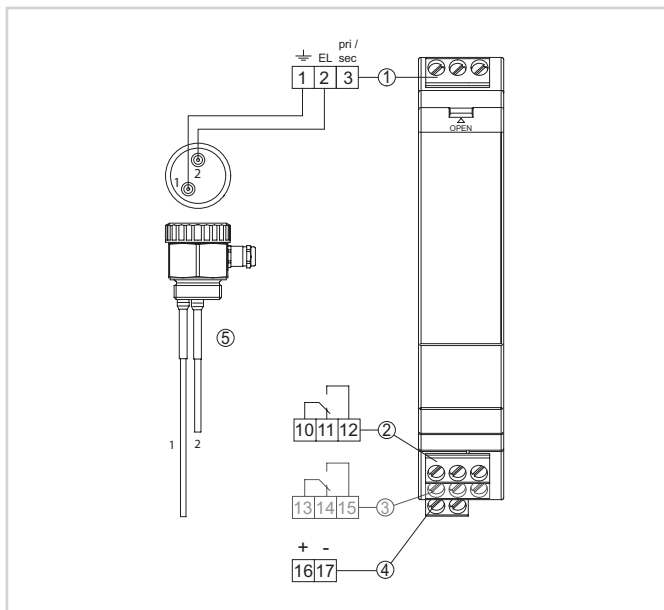
Wiring plan VEGATOR 131
