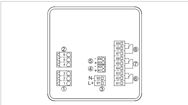
Wiring plan VEGAMET 342
