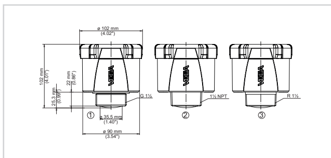
Dimensions VEGAPULS Air 41
