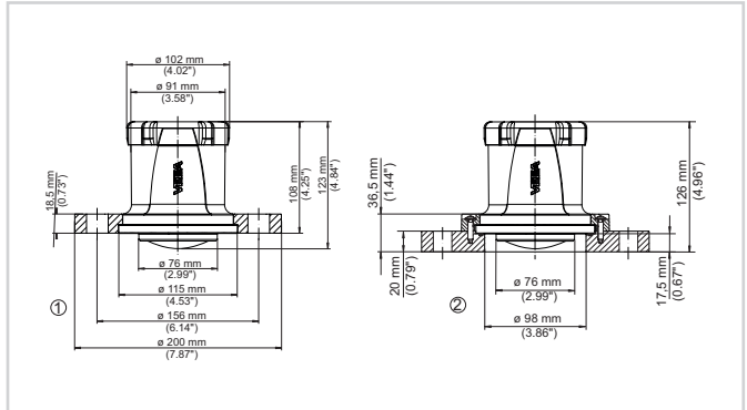
Dimensions VEGAPULS Air 42
