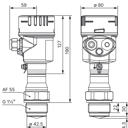
Variant G 1 1/2" PN 3 (DIN 3852-E)
