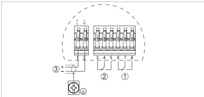
Wiring plan
