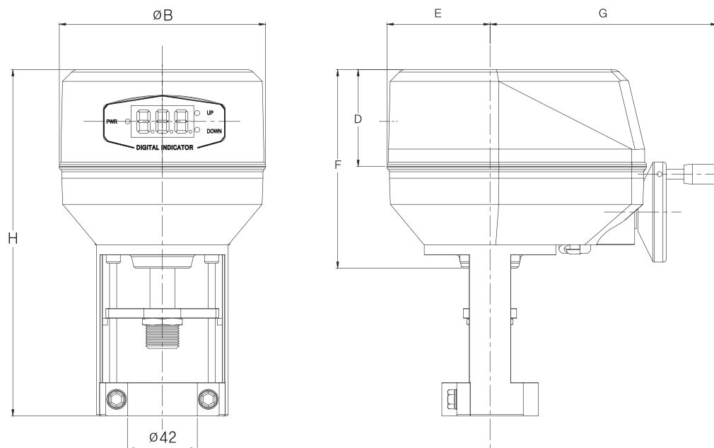
GEA-10PD
